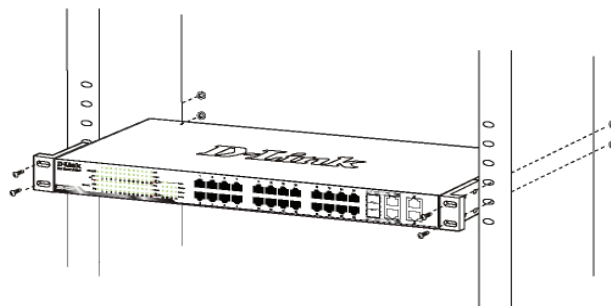
Рисунок 3. Установка коммутатора в стандартную стойку
