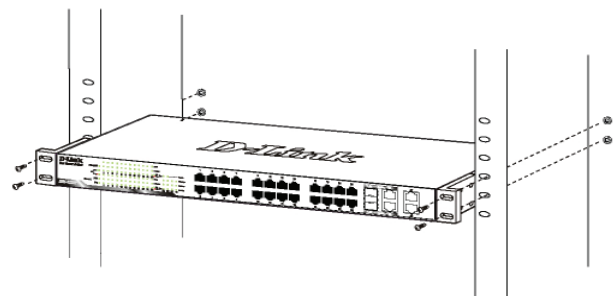
Abbildung 3: Switch im Standardrack installieren
