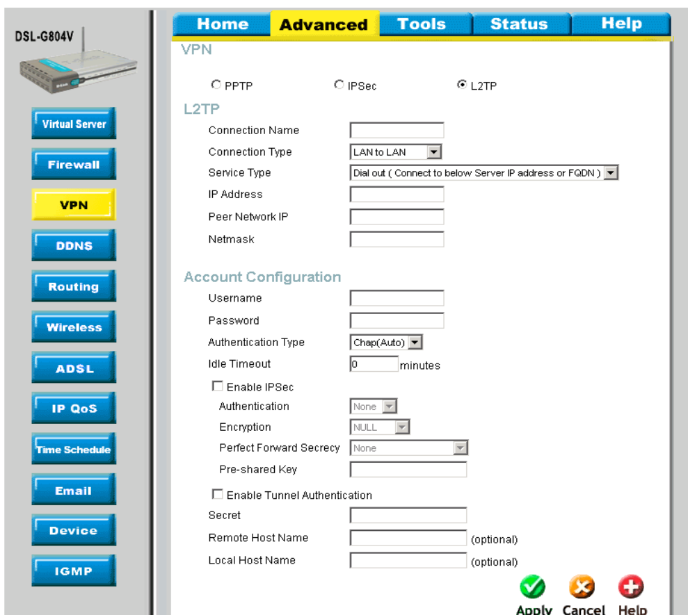
Figure 4-17. VPN – L2TP LAN to LAN
