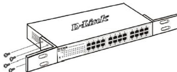
Рисунок 2. Крепление монтажных уголков
