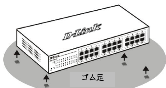
図1 ゴム足を取り付ける
